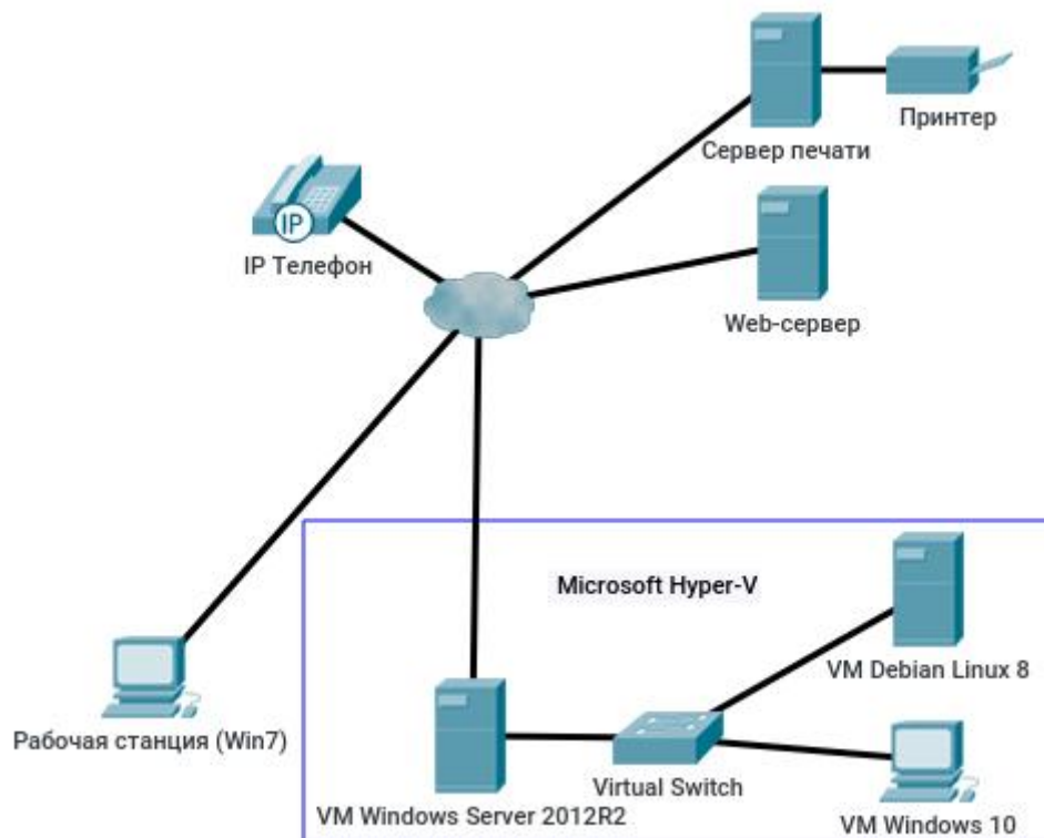
Рис.1. Топология сети
